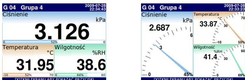
Rys. 7.159. Przykład prezentacji trzech kanałów z wyróżnieniem ciśnienia.
