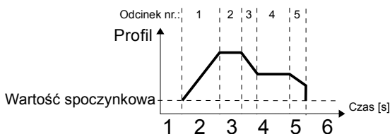
Rys.7.116. Przykładowy przebieg Profilu/timera
