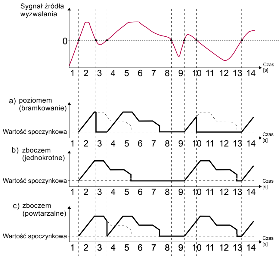
Rys.7.117. Przykładowe przebiegi wyjściowe Profilu zdefiniowanego na Rys.7.116 wyzwalanego sygnałem źródła wyzwalania dla Trybu wyzwalania: poziomem (bramkowanie) , zbczem (jednokrotne) , zbczem (powtarzalne)
