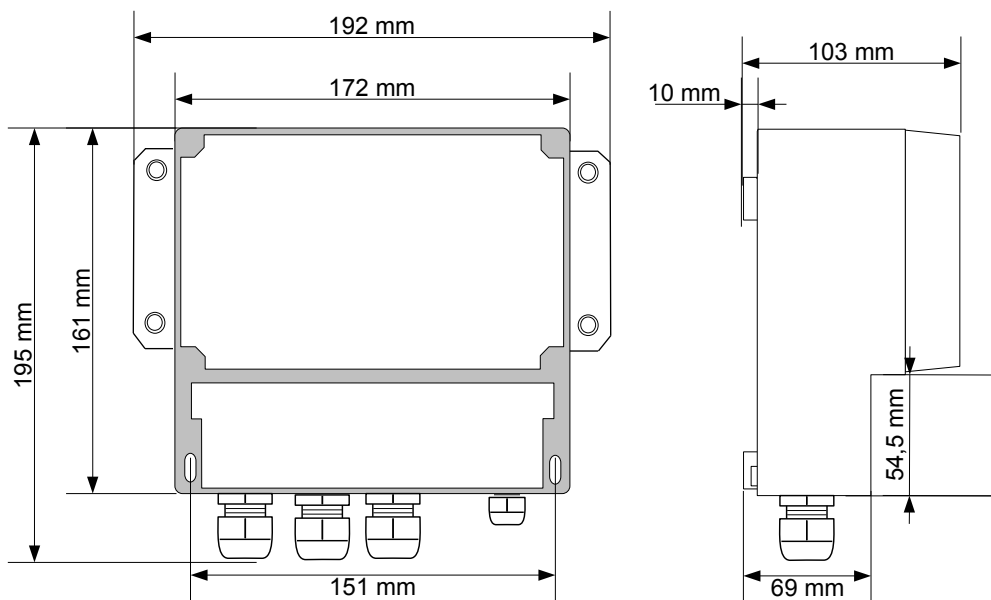
Rys. 4.3. Wymiary obudowy
