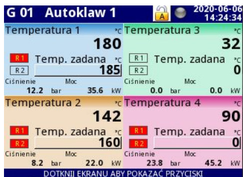
Rys. 7.162. Widok regulatorowy dla jednej grupy.
