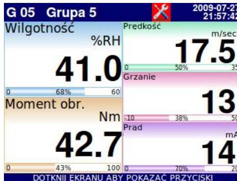
Rys. 7.47. Przykładowy widok ekranu z niezapisaną konfiguracją
