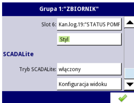
Rys. 7.151. Okno aktywacji trybu SCADALite
