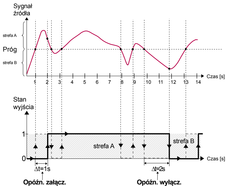
Rys. 7.97. Zasada pracy przekaźników wirtualnych dla przykładowych ustawień czasowych: Opóźn.załącz. = 1 sec., Opóźn.wyłącz. = 2 sec.
