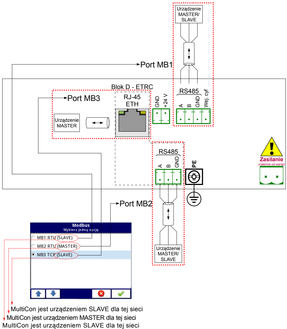
Rys. 7.63. Przykładowe podłączenie urządzenia MultiCon w sieci z podglądem skonfigurowanych portów Modbus
