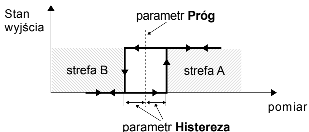
Rys. 7.94. Sterowanie jednoproęgowe przekaźnika wirtualnego
