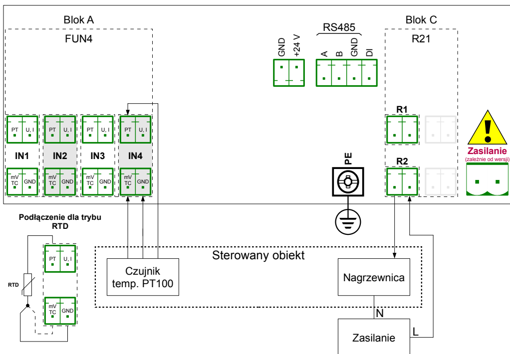
Rys. 7.105. Przykładowy sposób podłączenia do wejścia uniwersalnego w trybie RTD i wyjścia przekaźnikowego
