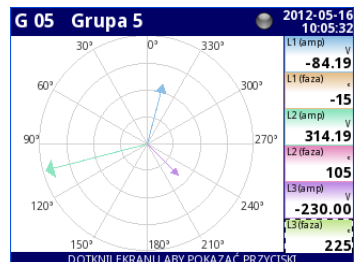
Rys. 6.12 Przykład Wykresów wskazowych
