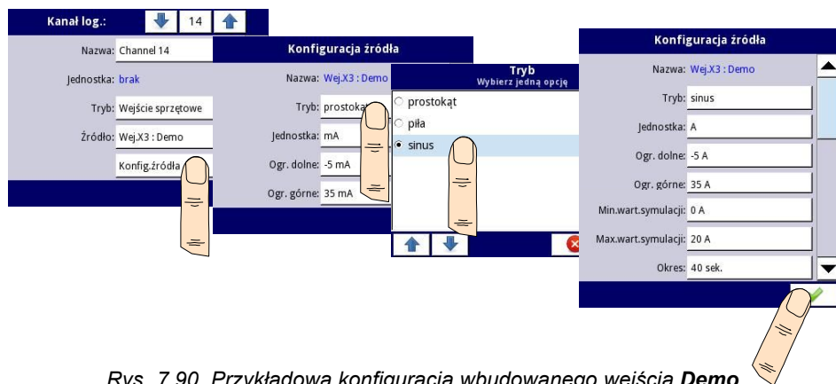
Rys. 7.90. Przykładowa konfiguracja wbudowanego wejścia Demo
