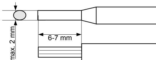
Rys. 4.2. Sposób odizolowania przewodów oraz wymiary końcówek kablowych
