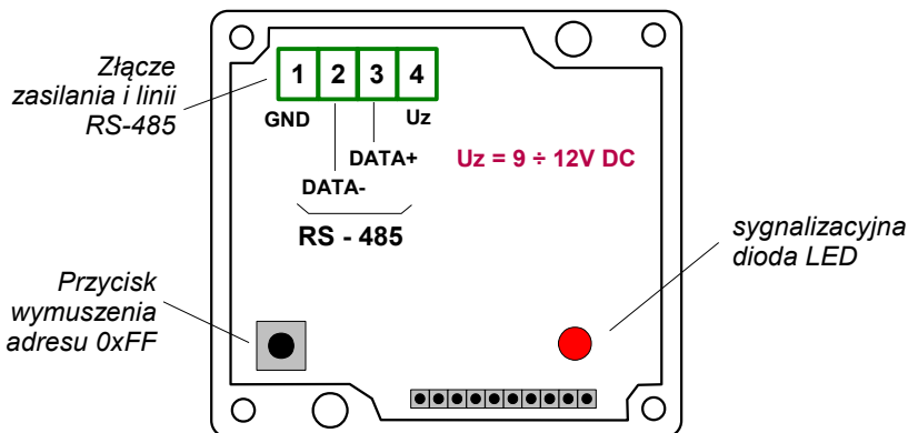
Rys. 4.3. Rozmieszczenie złącz wewnątrz obudowy
